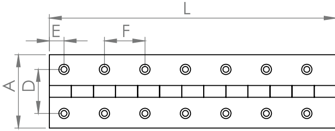
Delik Dizilişi Düz Straight Hole Array
