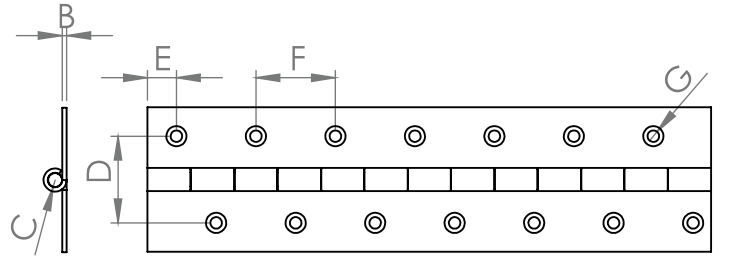
Delik Dizilişi Çapraz Diagonal Hole Array
